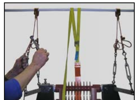
16. Opphengsliner forspennes.
